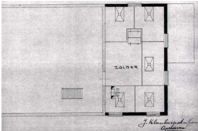
Gedeelten van de bouwtekening behorend bij het schrijven van 22 januari 1923, respectievelijk de plattegrond van de in te richten maalderij en de zolderverdieping. Links op de plattegrond is het gedeelte van de latere winkel. Ook de verhoogde stoep buiten staat aangegeven.
